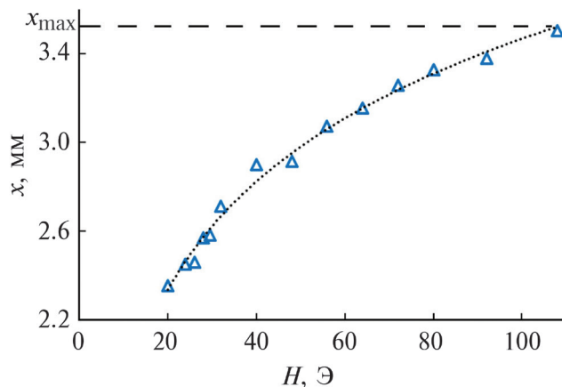
Рис. 4. Зависимость установившегося равновесного положения доменных границ при ее смещении вдоль клина Pt после приложения отдельных серий импульсов магнитного поля с фиксированной амплитудой в каждой серии.
